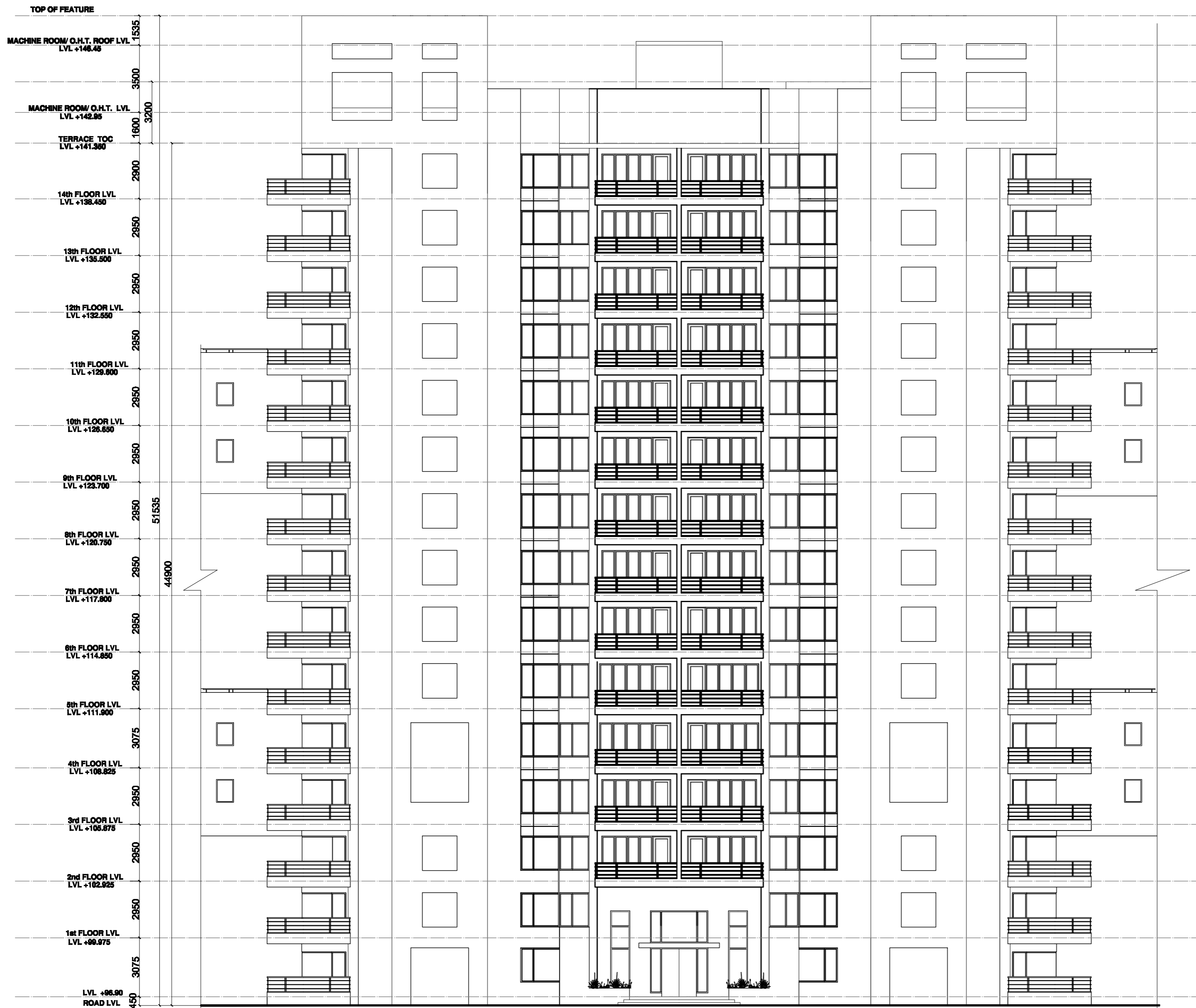
FRONT ELEVATION D5
